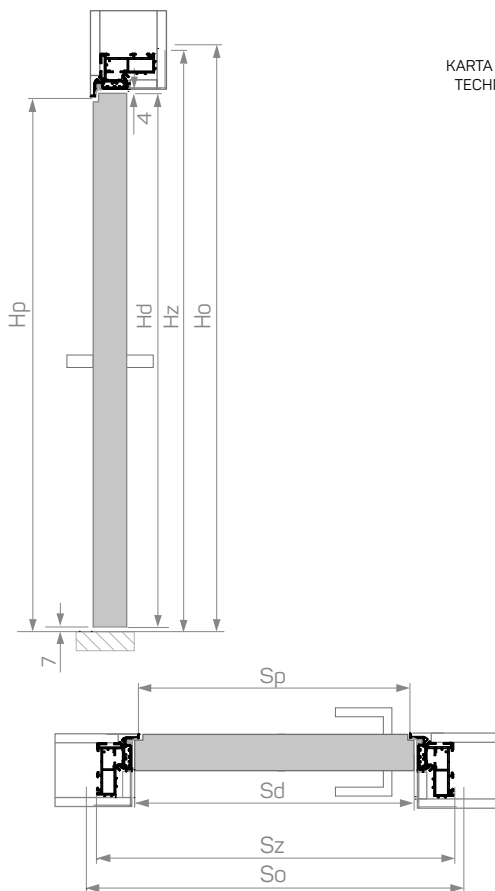
DRZWI PRZECIWPÓŻAROWE WEWNĘTRZNE - SKRZYDŁO DREWNIANE INTERNAL FIRE RESISTANT DOORS - WOODEN DOOR LEAF
