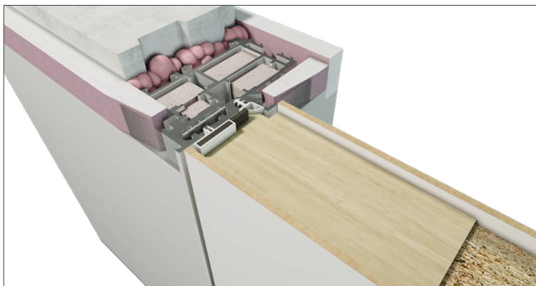
DRZWI PRZECIWPÓŻAROWE ZEWNĘTRZNE - SKRZYDŁO DREWNIANE EXTERNAL FIRE RESISTANT DOORS - WOODEN DOOR LEAF
