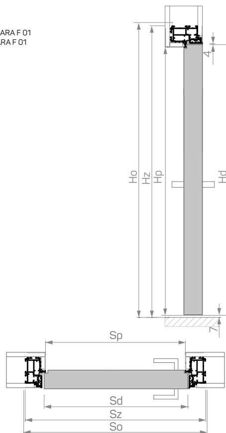
DRZWI PRZECIWPÓŻAROWE WEWNĘTRZNE - SKRZYDŁO DREWNIANE INTERNAL FIRE RESISTANT DOORS - WOODEN DOOR LEAF
